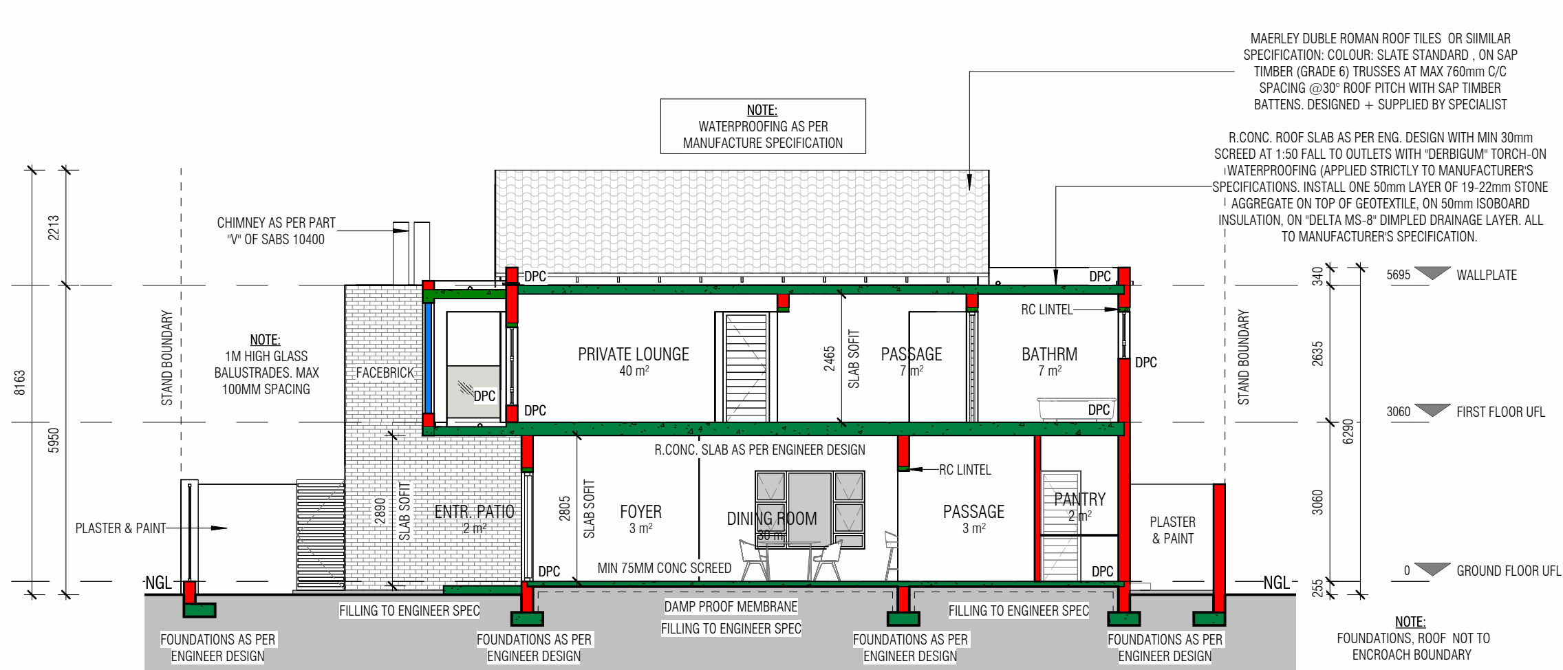
B SECTION B-B 1 : 100
