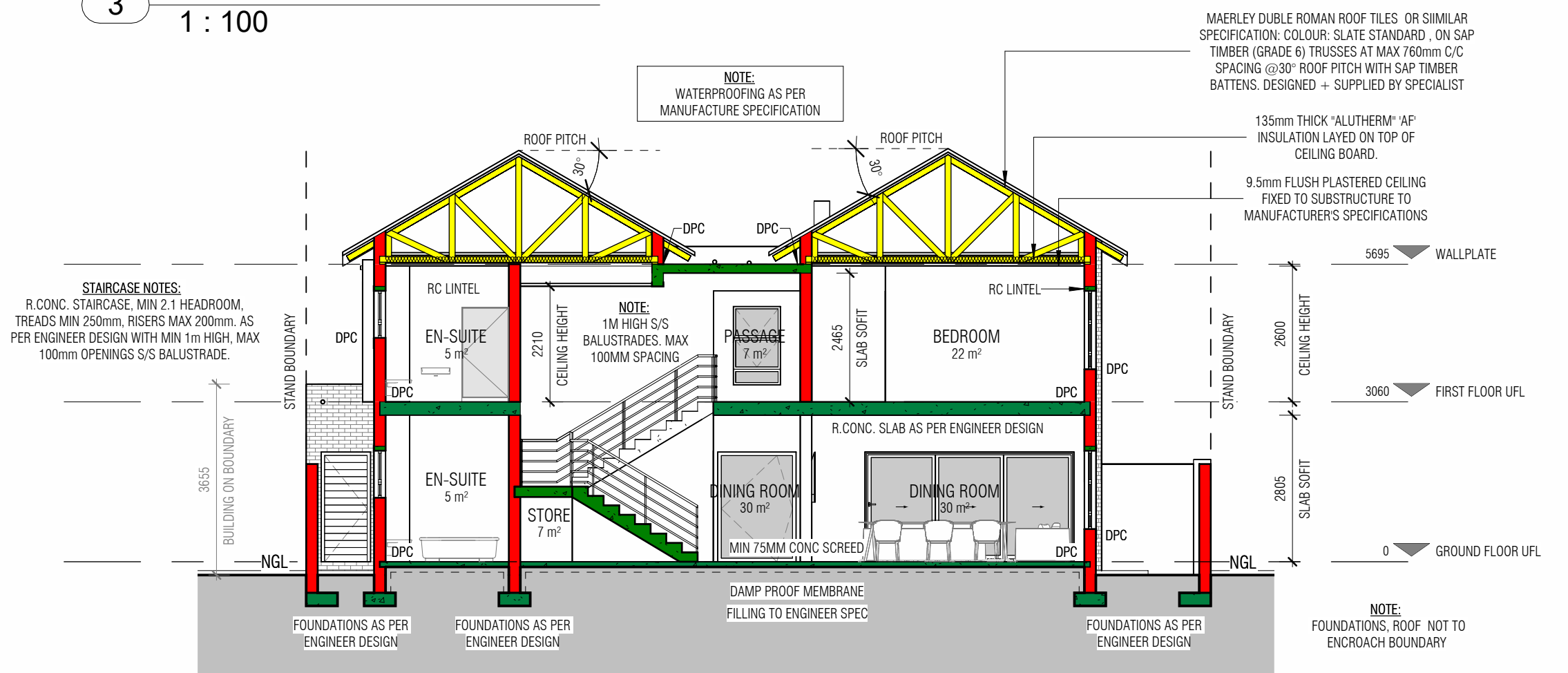
A SECTION A-A 1 : 100
